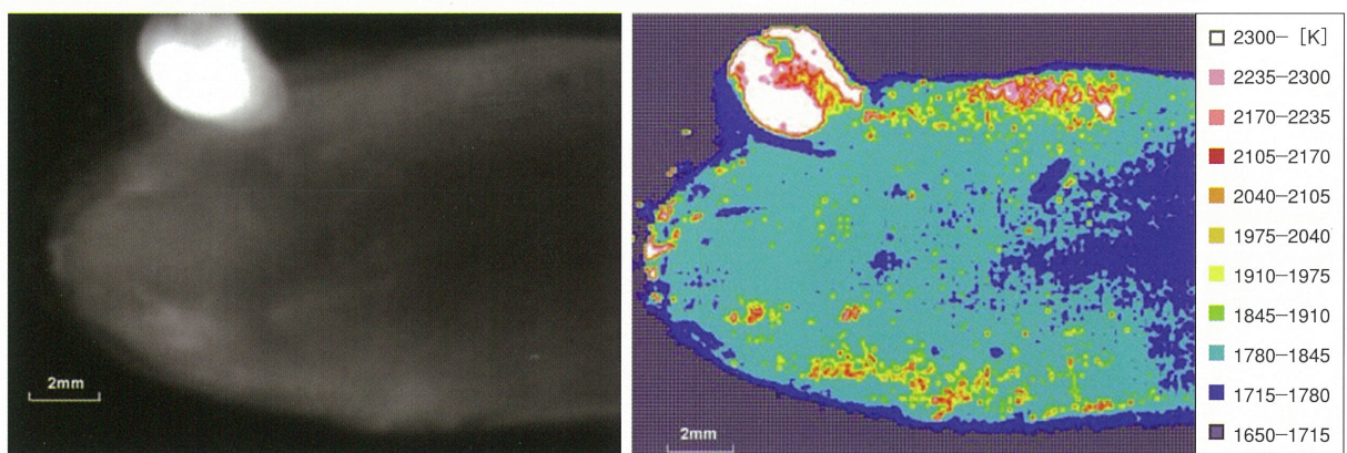
本文記事 図10 炭酸ガスアーク溶接における溶融池の表面温度
