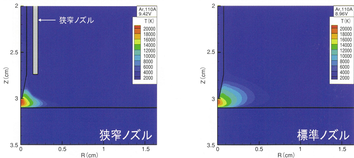
本文記事 図13 数値計算シミュレーションの見える化による狭窄ノズルの効果
