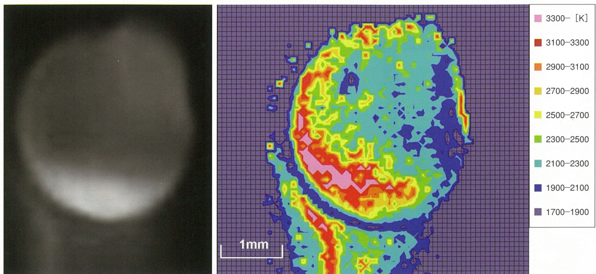
本文記事 図9 炭酸ガスアーク溶接における溶滴の表面温度
